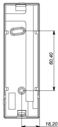
Рис 9. Разметка крепежных
