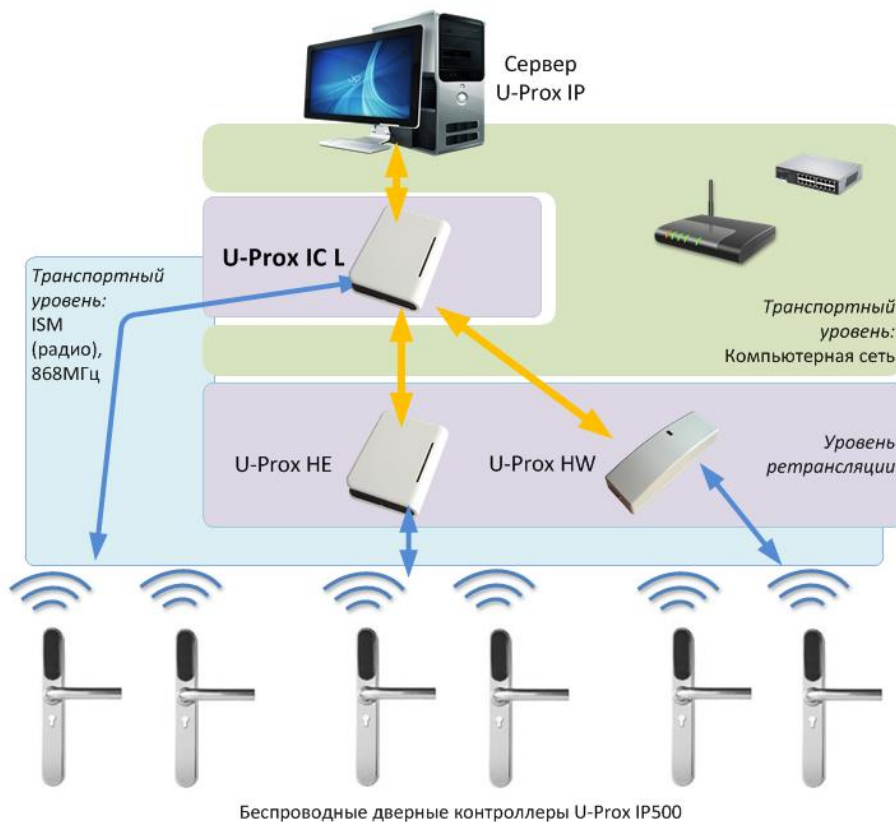
Рис 6. Построение системы беспроводных замков
